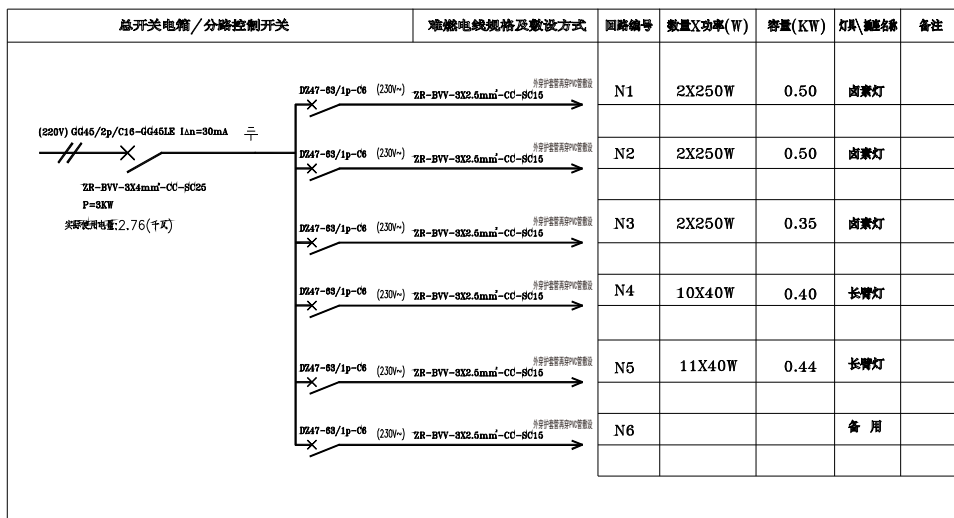
配电系统图
